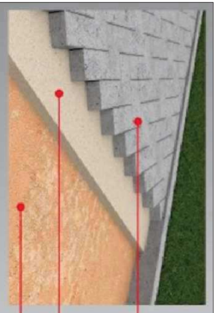
PISO INTER TRAVADO DE CONCRETO (8 cm) CAMADA DE ASSENTAMENTO - AREIA (10 cm) TERRENO NIVELADO E COMPACTADO
