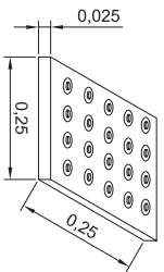
DEFINIÇÃO PISO TÁTIL SEM ESCALA
