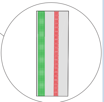
DETALHE PISO TÁTIL (PASSEIO PÚBLICO) SEM ESCALA
