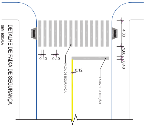
DETALHE DE FAIXA DE SEGURANÇA ELEVADA (altura 10,0 cm) SEM ESCALA
