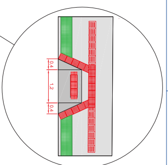
DETALHE RAMPA CADIRANTES SEM ESCALA
